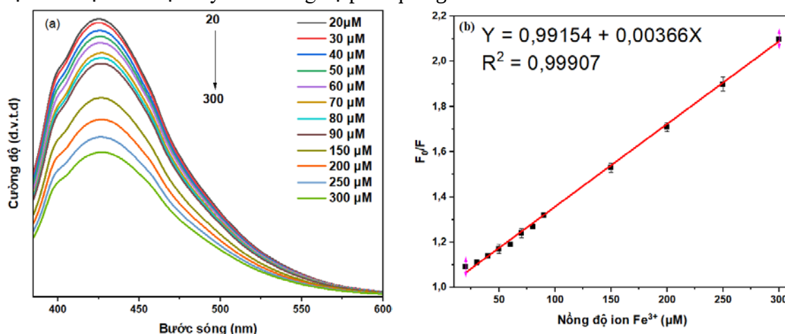
Hình 6. (a) Phổ phát quang của dung dịch CNPs chứa ion Fe^{3+} ứng với các giá trị nồng độ khác nhau ( \lambda_{ex} = 350 nm). (b) Các giá trị nồng độ của ion Fe^{3+} trong khoảng 20 \mu M đến 300 \mu M được biểu diễn theo phương trình Stern-Volmer dựa vào tỷ số F_0/F ( \lambda_{ex} = 350 nm)
