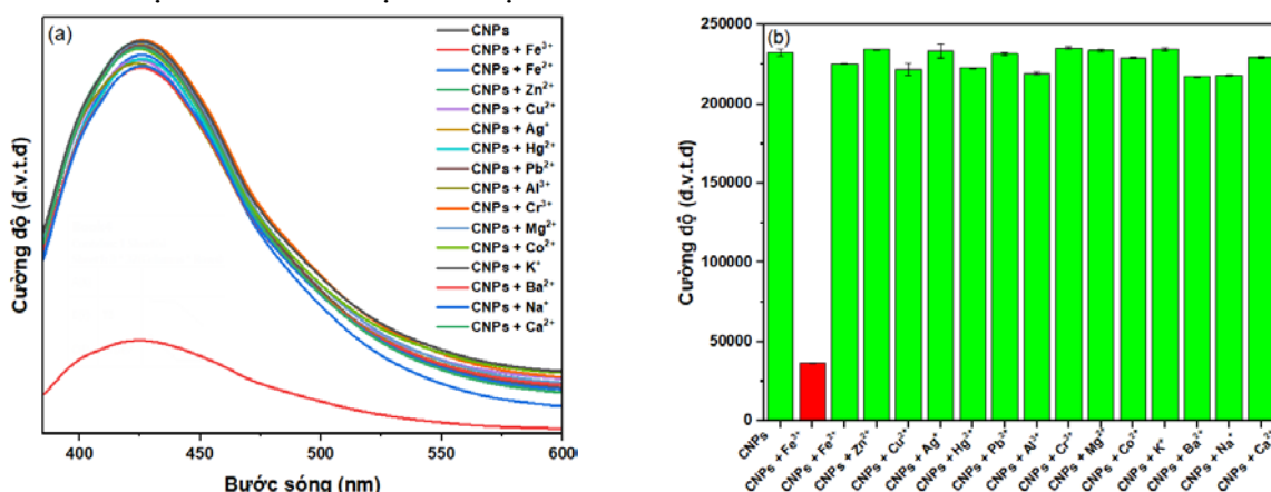
Hình 5. (a) Phổ phát quang của dung dịch CNPs khi có và không có mặt các ion kim loại ( \lambda_{ex} = 350 nm). (b) Cường độ phát quang tại vị trí bước sóng 426 nm của CNPs khi có và không có mặt các ion kim loại
