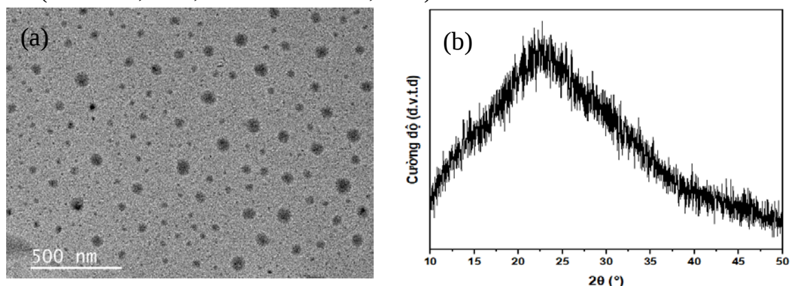
Hình 2. (a) Ảnh TEM của CNPs với thanh định cỡ 500 nm (b) Giản đồ nhiễu xạ tia X của CNPs
