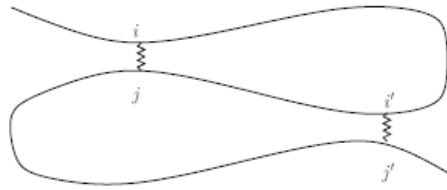
Hình 3. Cấu trúc RNA có nút thắt (pseudoknotted)
